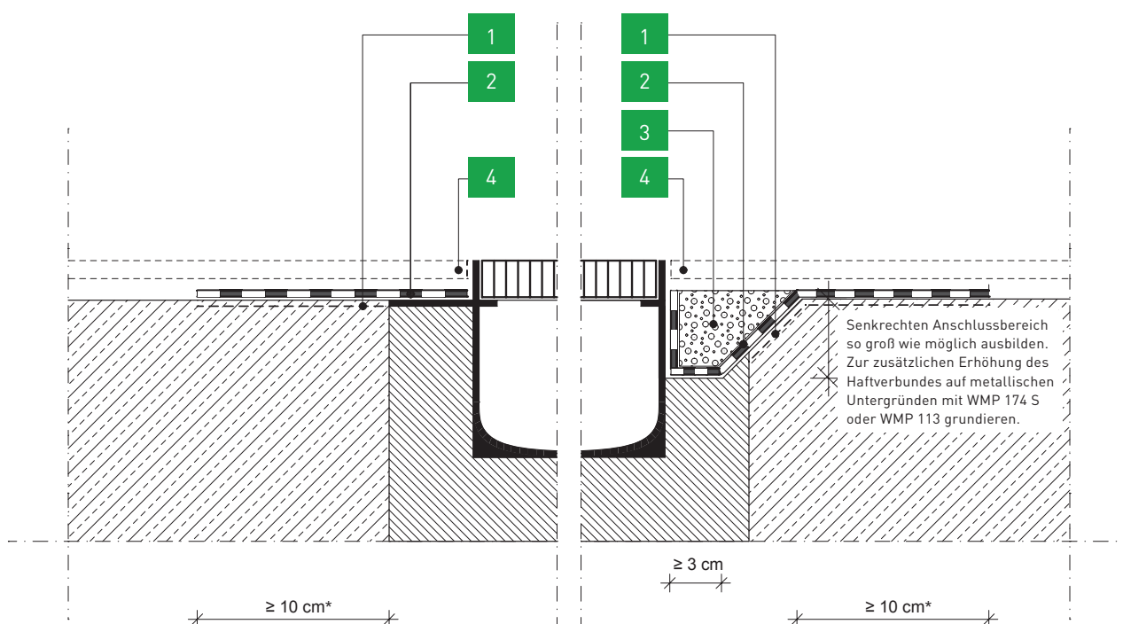
mit Anschlussflansch
